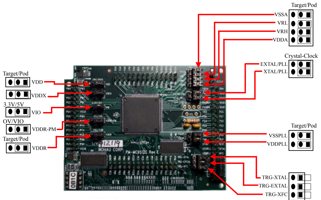
MC9S12E128 CPU Module
